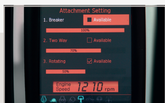
Accessoires : réglage du débit du circuit hydraulique auxiliaire
